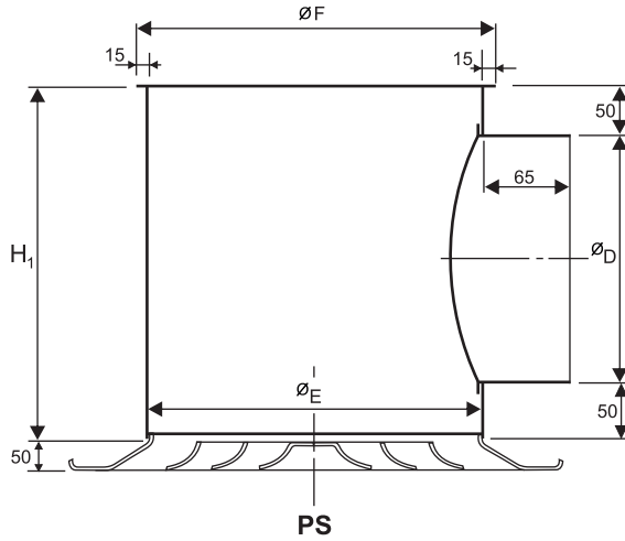
PS Yan girişli plenum / Plenum box with side entry
