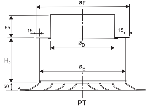
PT Üstten girişli plenum / Plenum box with top entry
