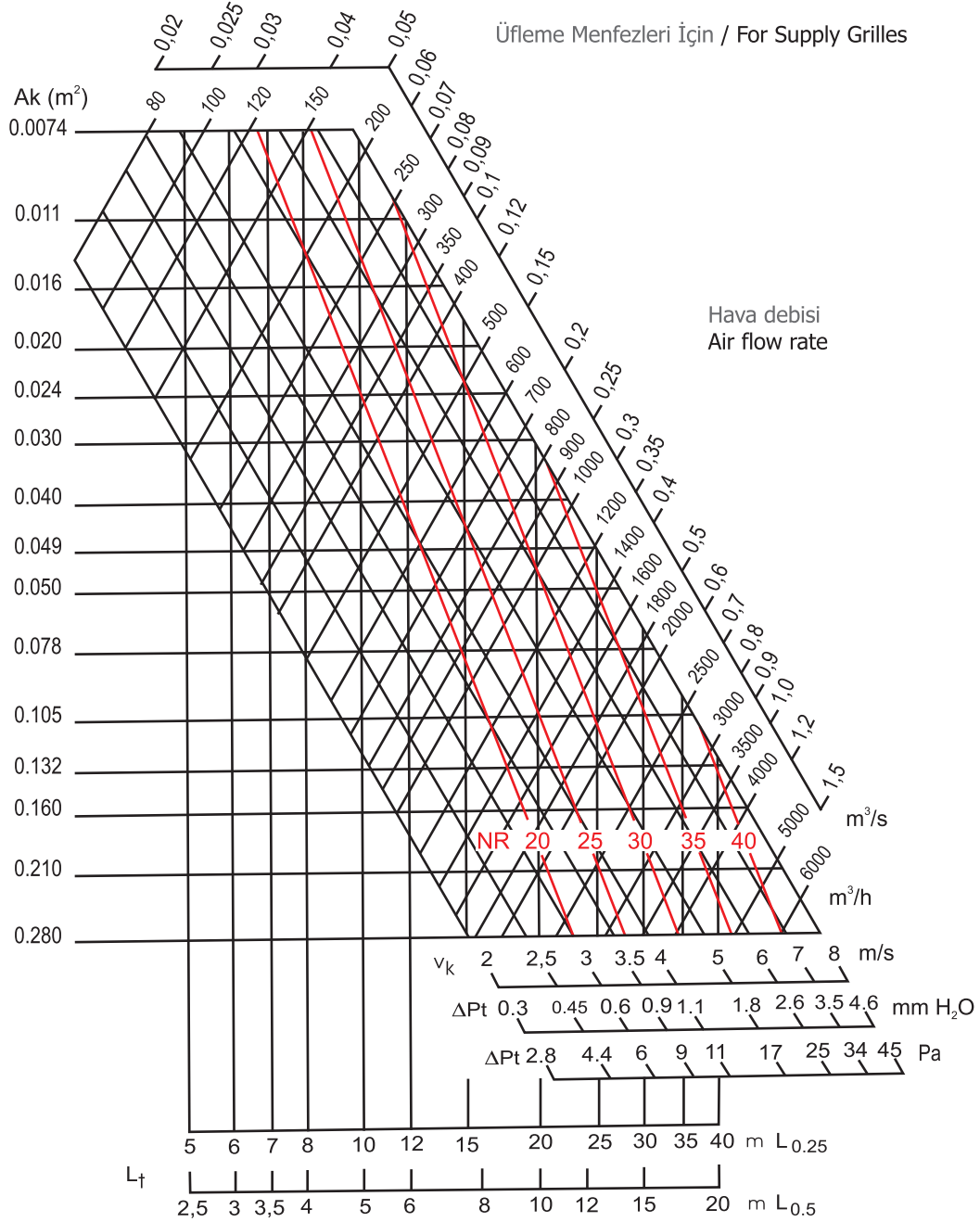
Düzeltilme Faktörleri / Correction Factors
