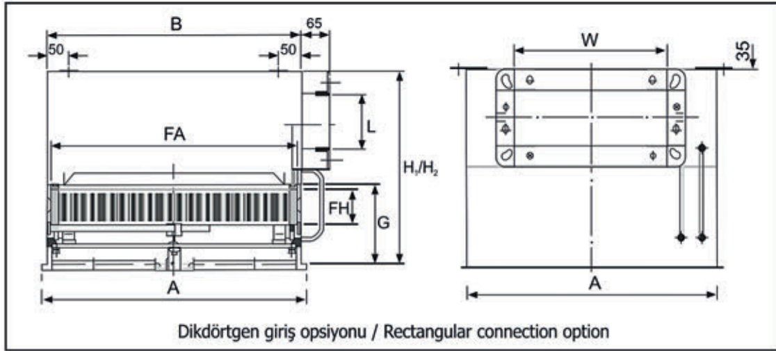
Plenum kutu ve filtre ölçüleri / Plenum box & filter dimensions
